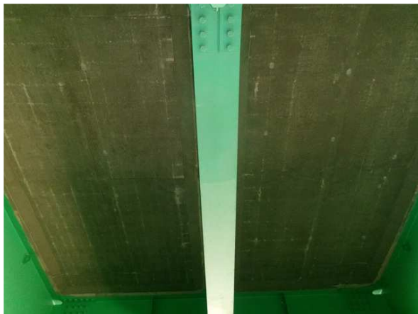
바닥판하면 전경
