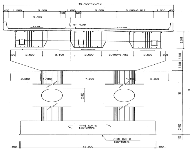
<횡단면도>
